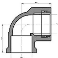
Joelho 90° Soldável e Com Bucha de Latão
